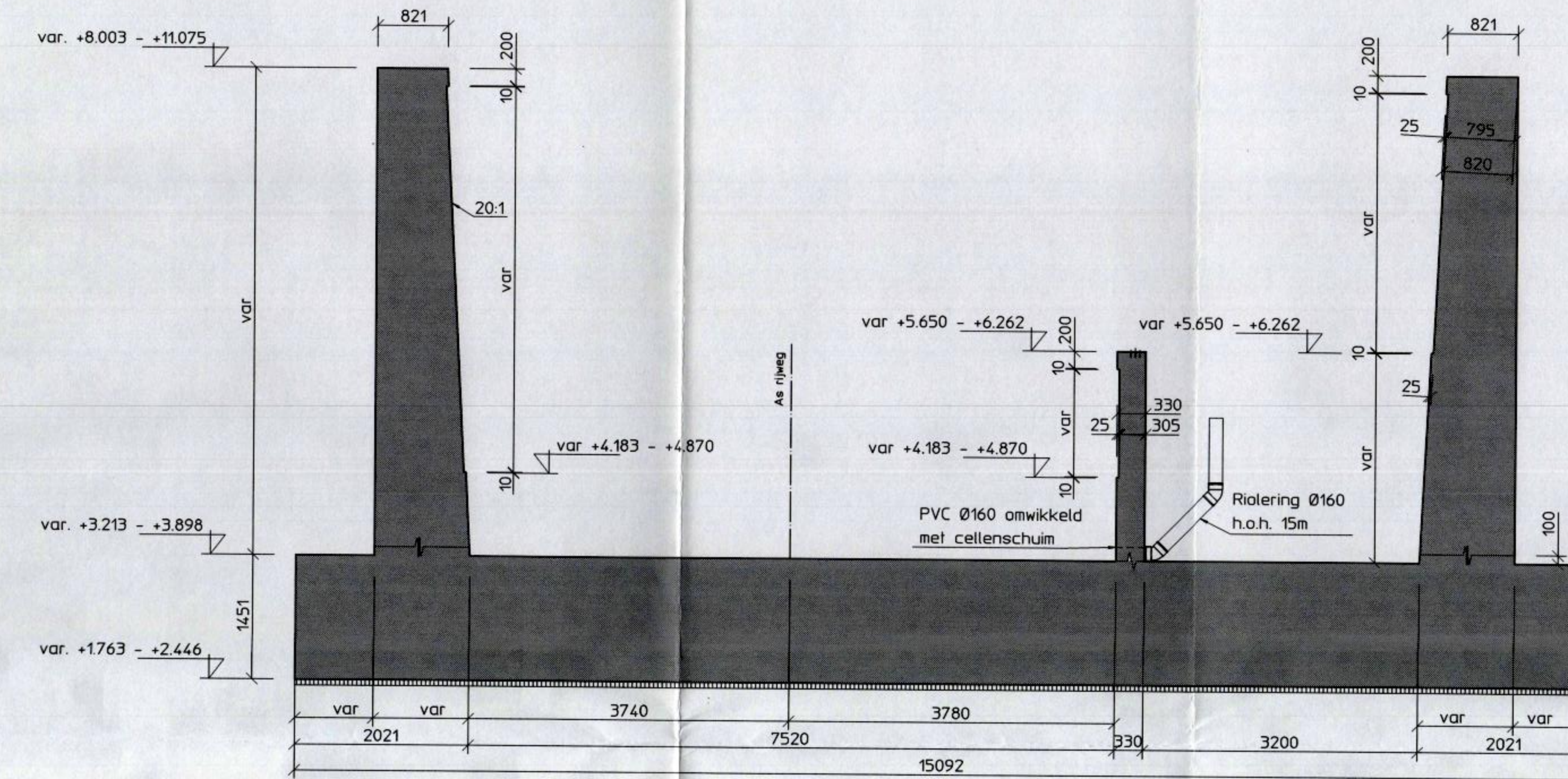
Doorsnede E
