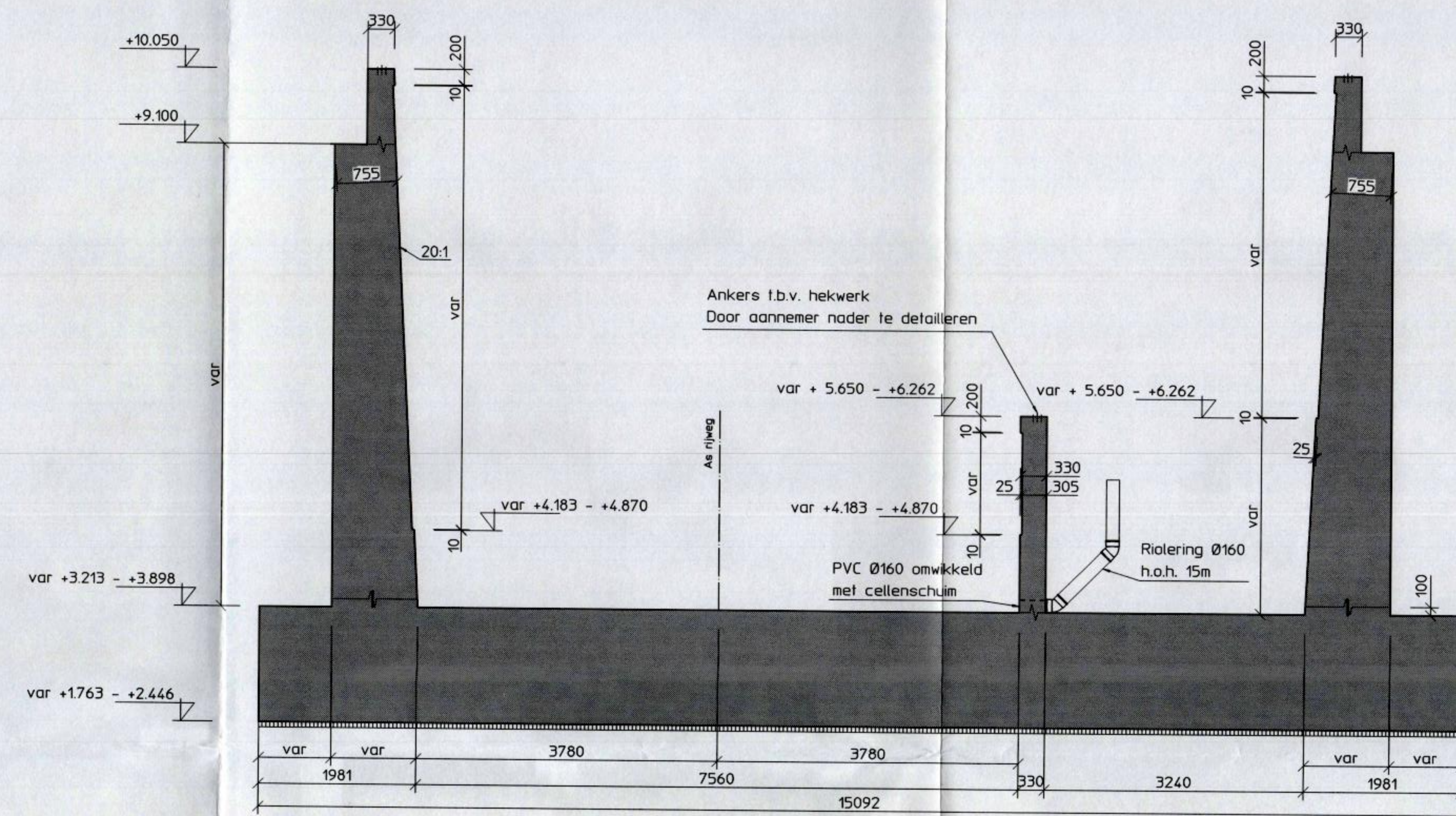
Doorsnede D
