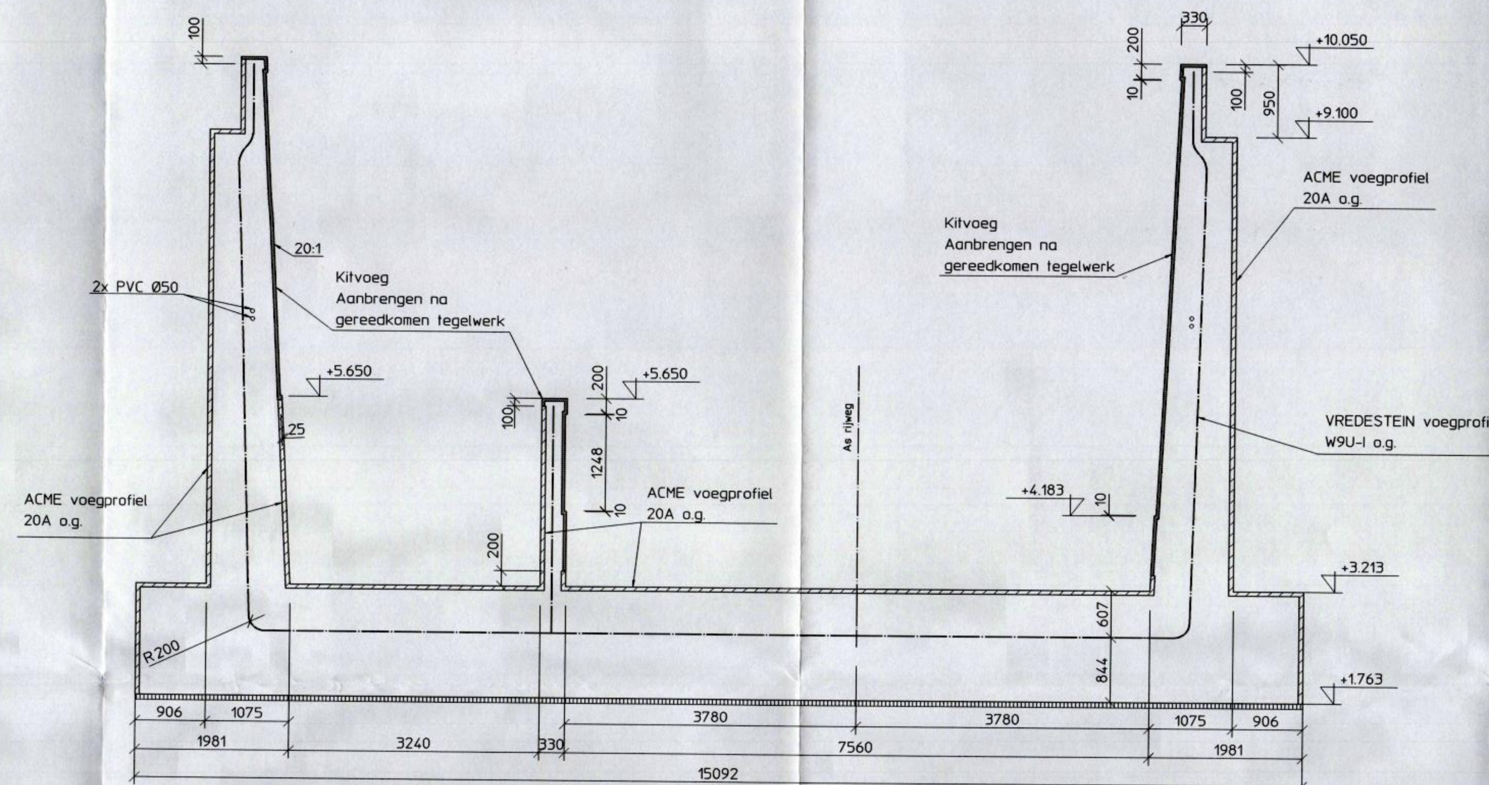
Aanzicht F
