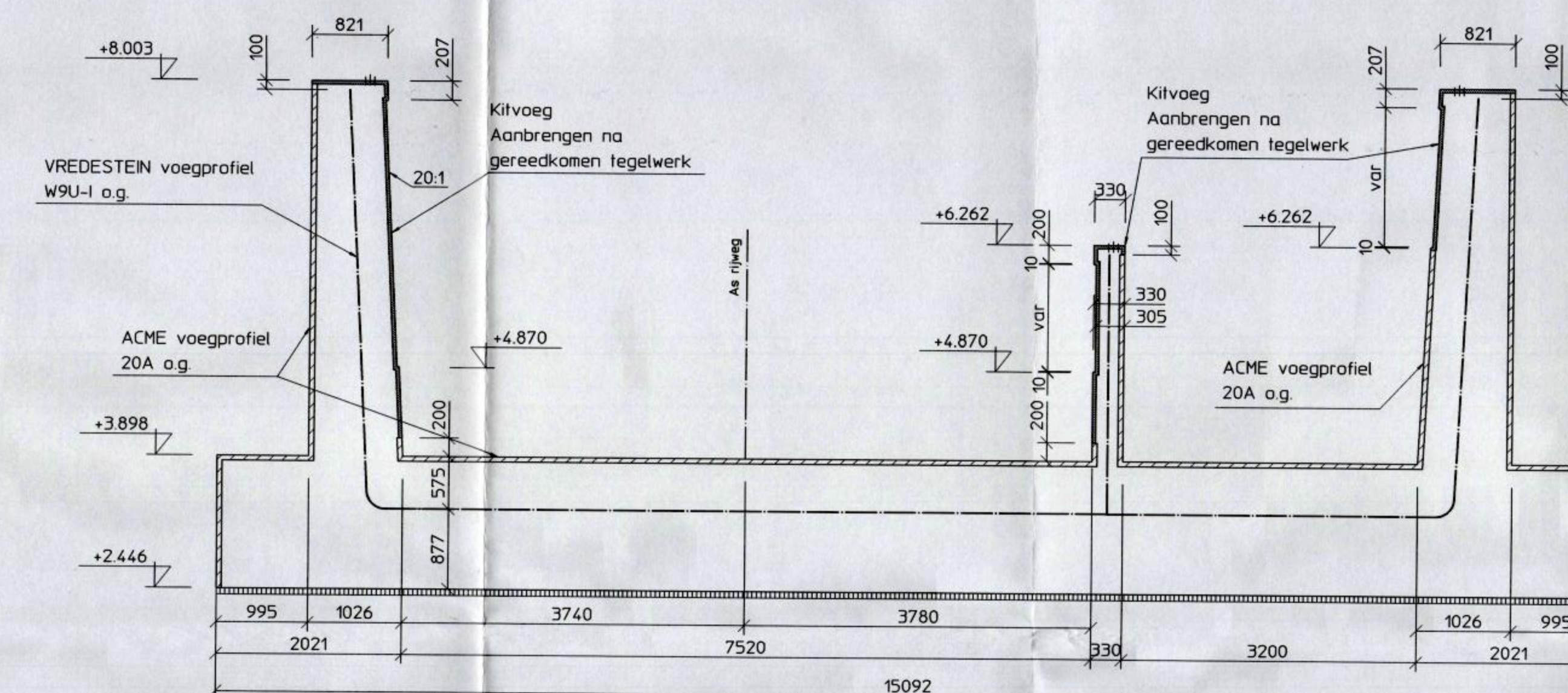
Aanzicht G
